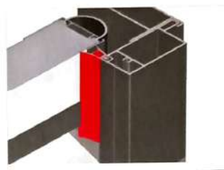
Joint tubulaire à lèvre EPDM côté fermeture
