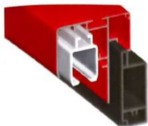
Précadre avec profil de rail monobloc laqué noir
