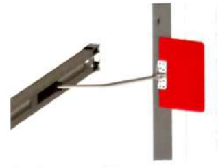
Plaque renfort pour liaison du bras moteur
