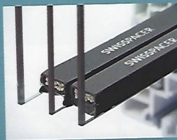
Intercalaire présenté dans une version triple vitrage
