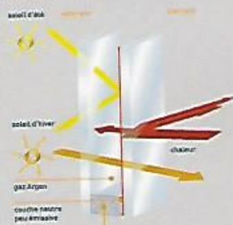
Isolation thermique renforcée de base
