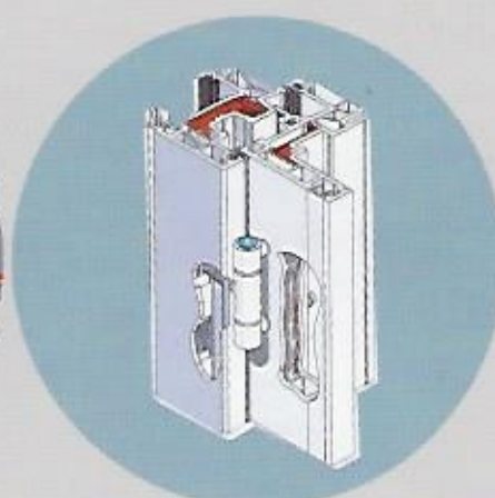
Ferrage triple broche Résistance à l'arrachement (jusqu'à 700 kg)
